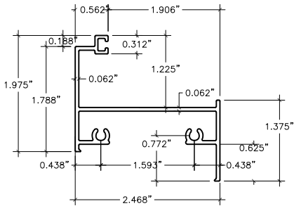
2 FRAME JAMB
